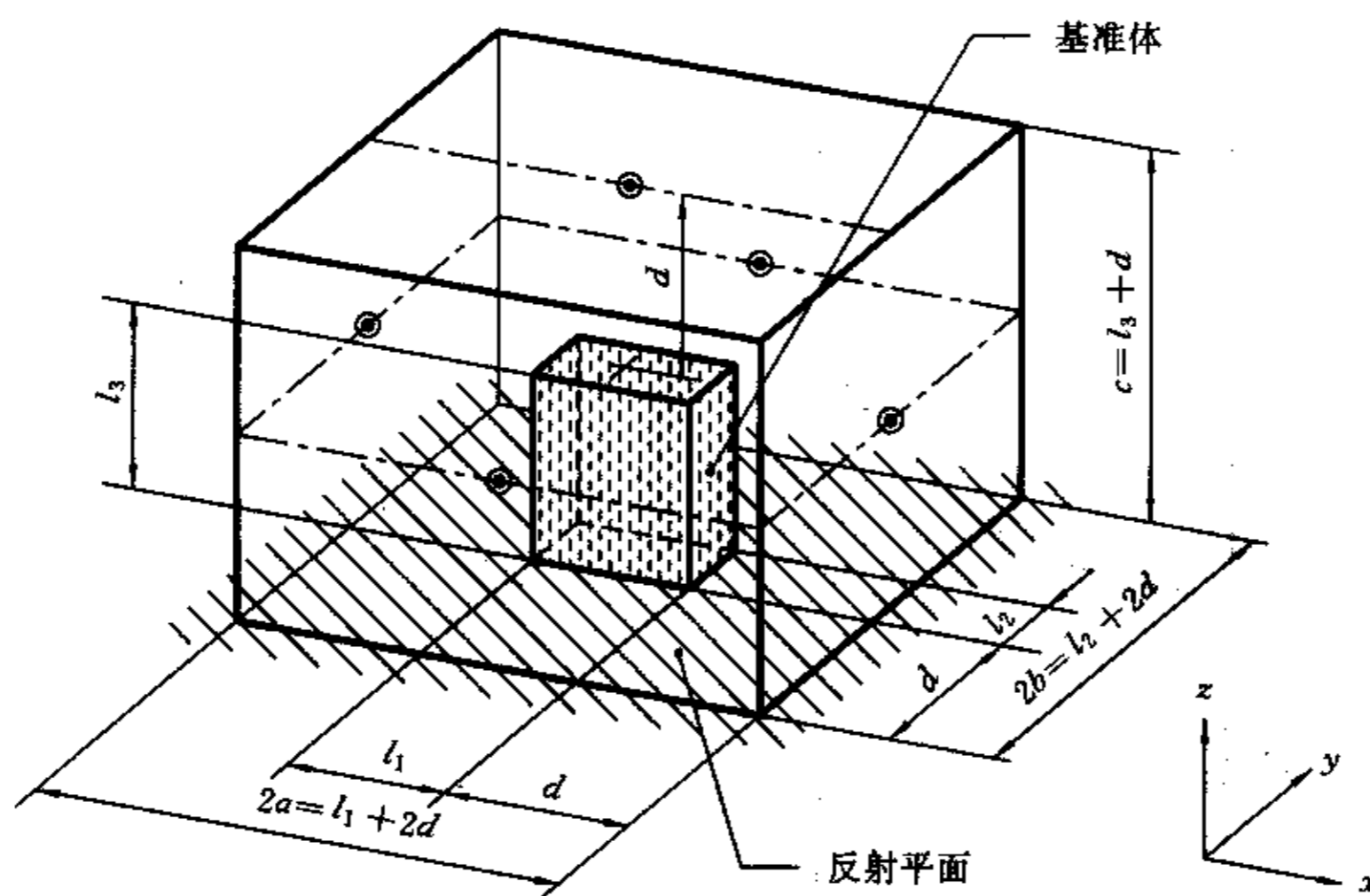
图 C2 小型机器测量表面和传声器位置示例 ( l_1 \leq d, l_2 \leq d, l_3 \leq 2d, d 为测量距离,一般为 1 m)
