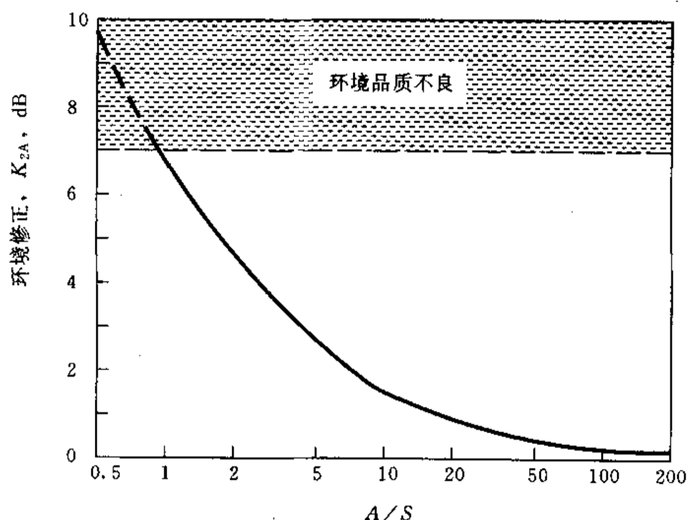
图 A1 环境修正 K_{2A}
