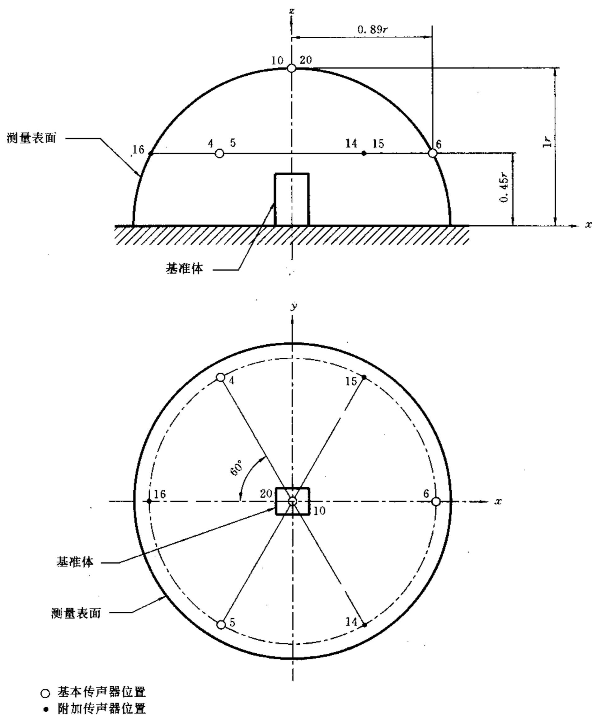
图 B2 半球表面上的传声器阵列
