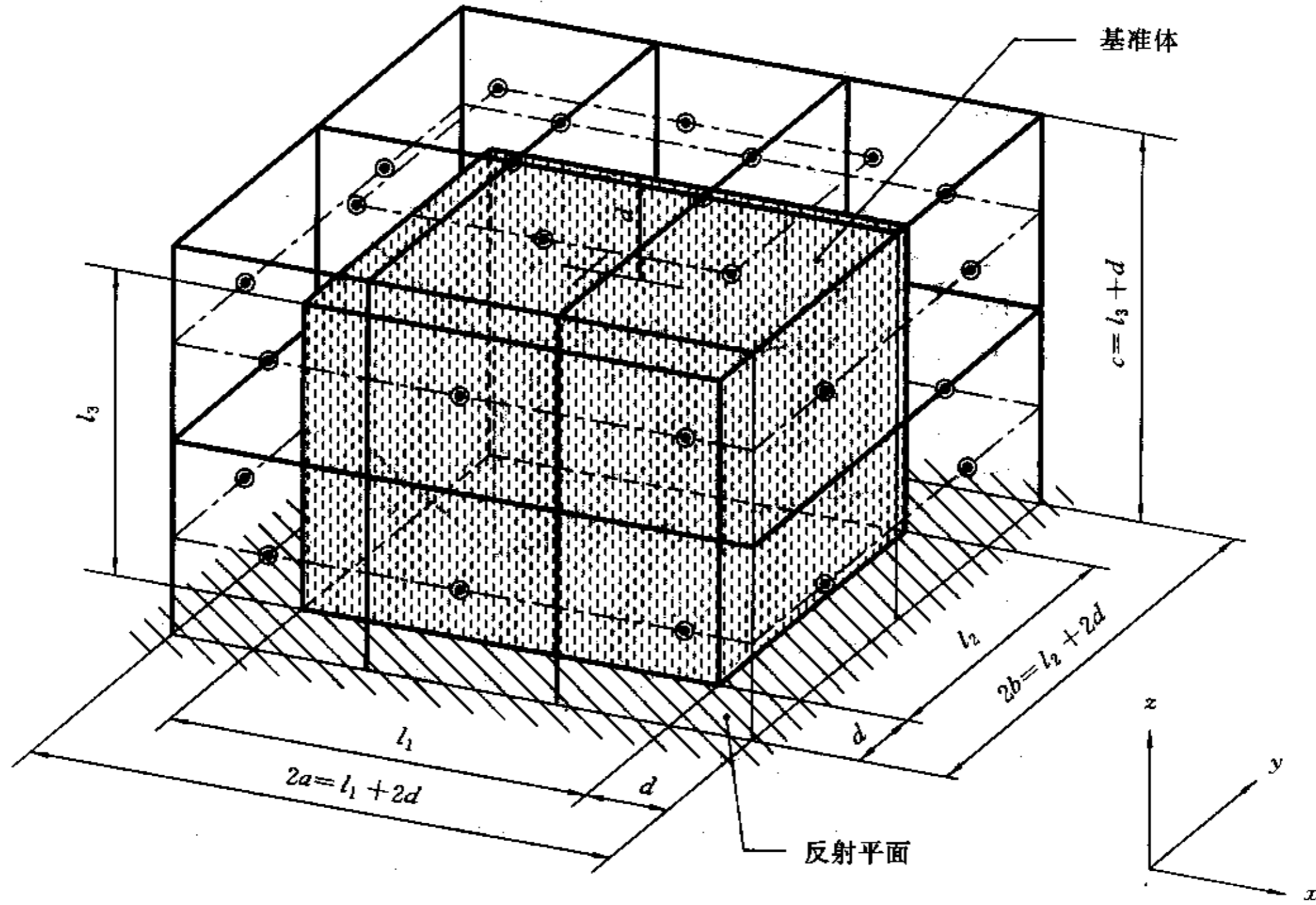
图 C6 大型机器测量表面和传声器位置示例 (4d < l_1 \leq 7d, d < l_2 \leq 4d, 2d < l_3 \leq 5d)
