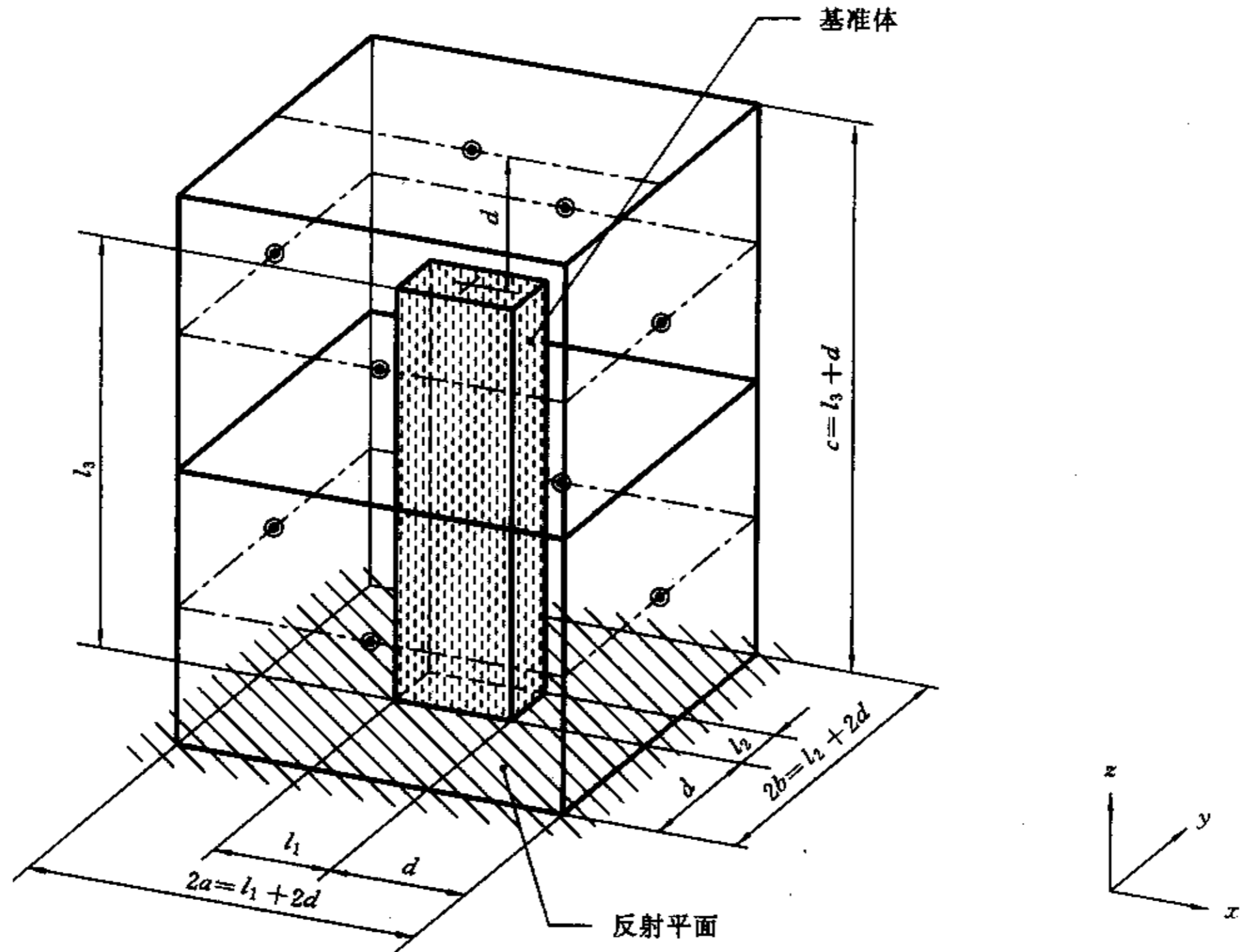
图 C3 小底座高机器测量表面和传声器位置示例 (l_1 \leq d, l_2 \leq d, 2d < l_3 \leq 5d)
