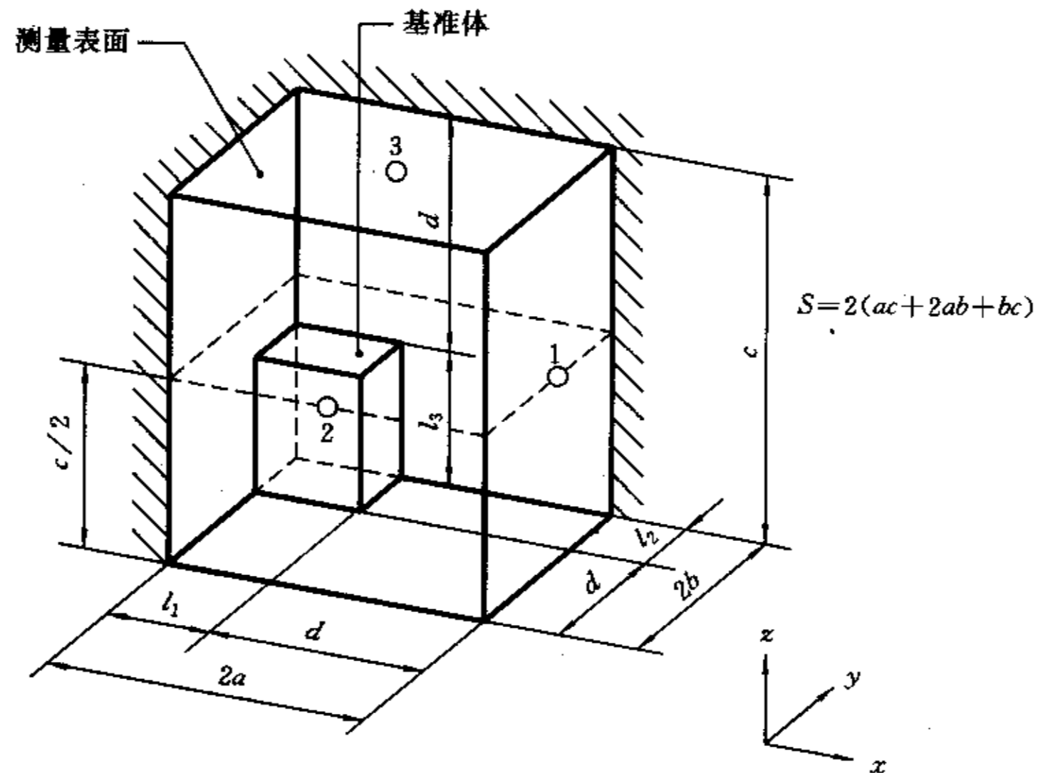
图 C8 地立设备靠两面墙放置,有三个传声器位置的平行六面体测量表面
