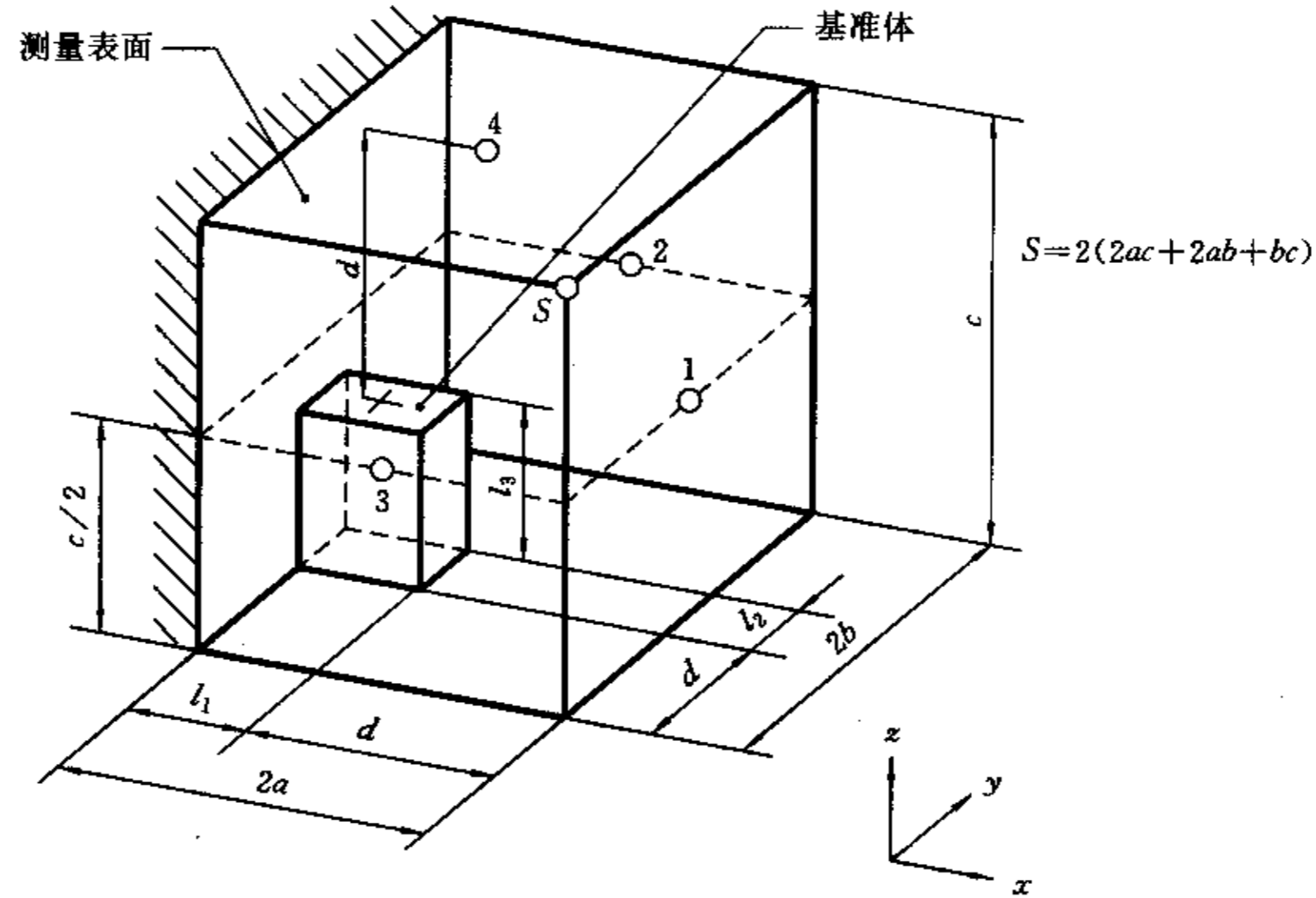
图 C7 地立设备靠一面墙放置,有四个传声器位置的平行六面体测量表面
