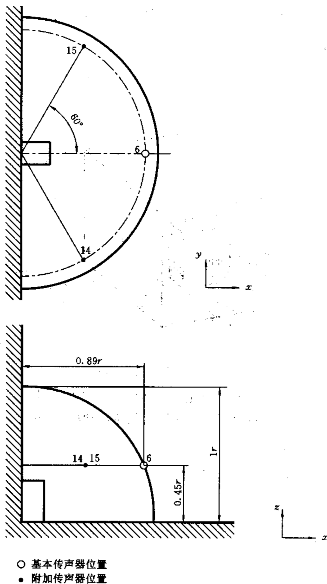
图 B3 基准体紧靠两个反射面的局部球形测量表面与传声器位置平面图
