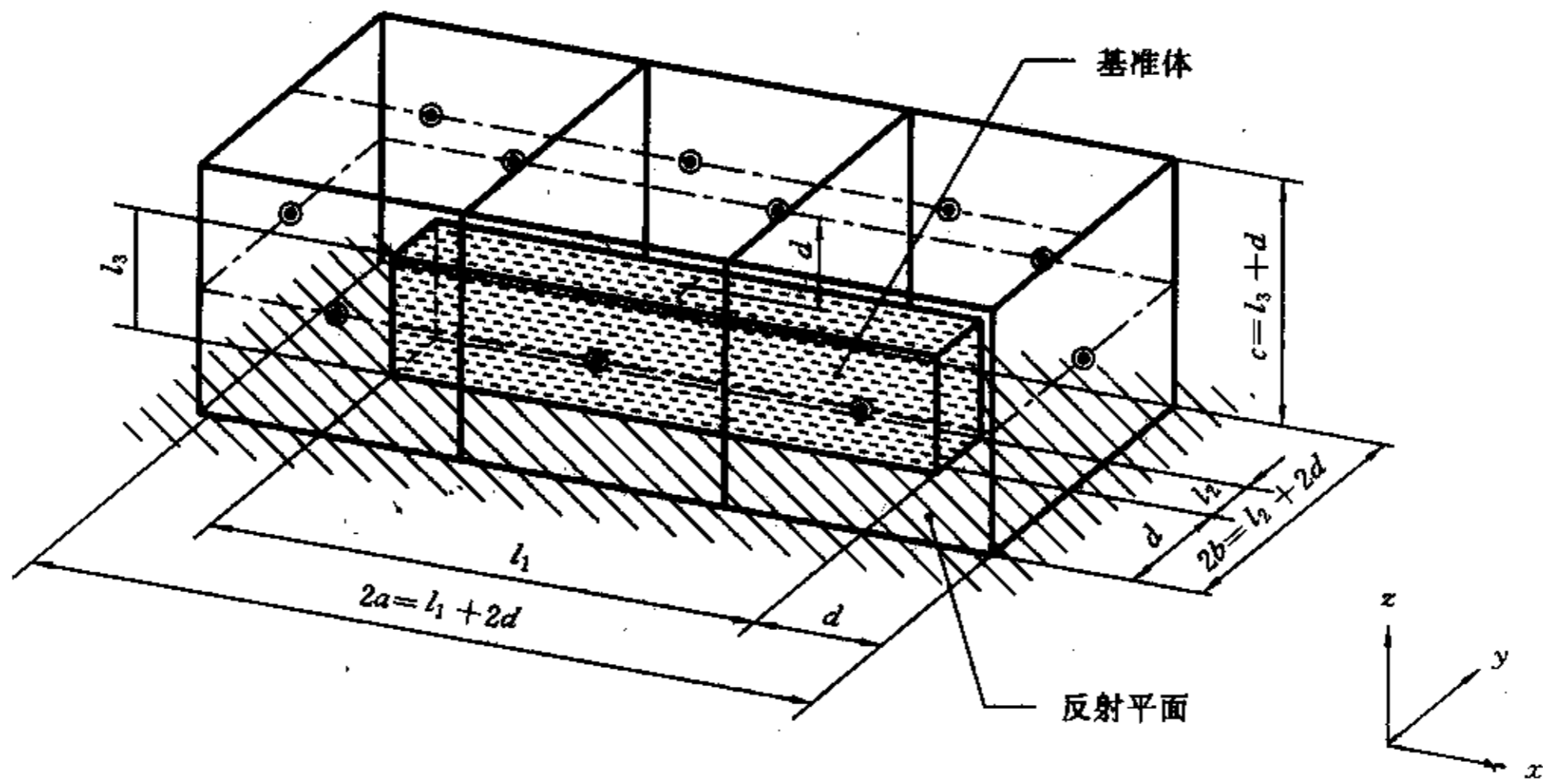
图 C4 长型机器测量表面和传声器位置示例 (4d < l_1 \leq 7d, l_2 \leq d, l_3 \leq 2d)
