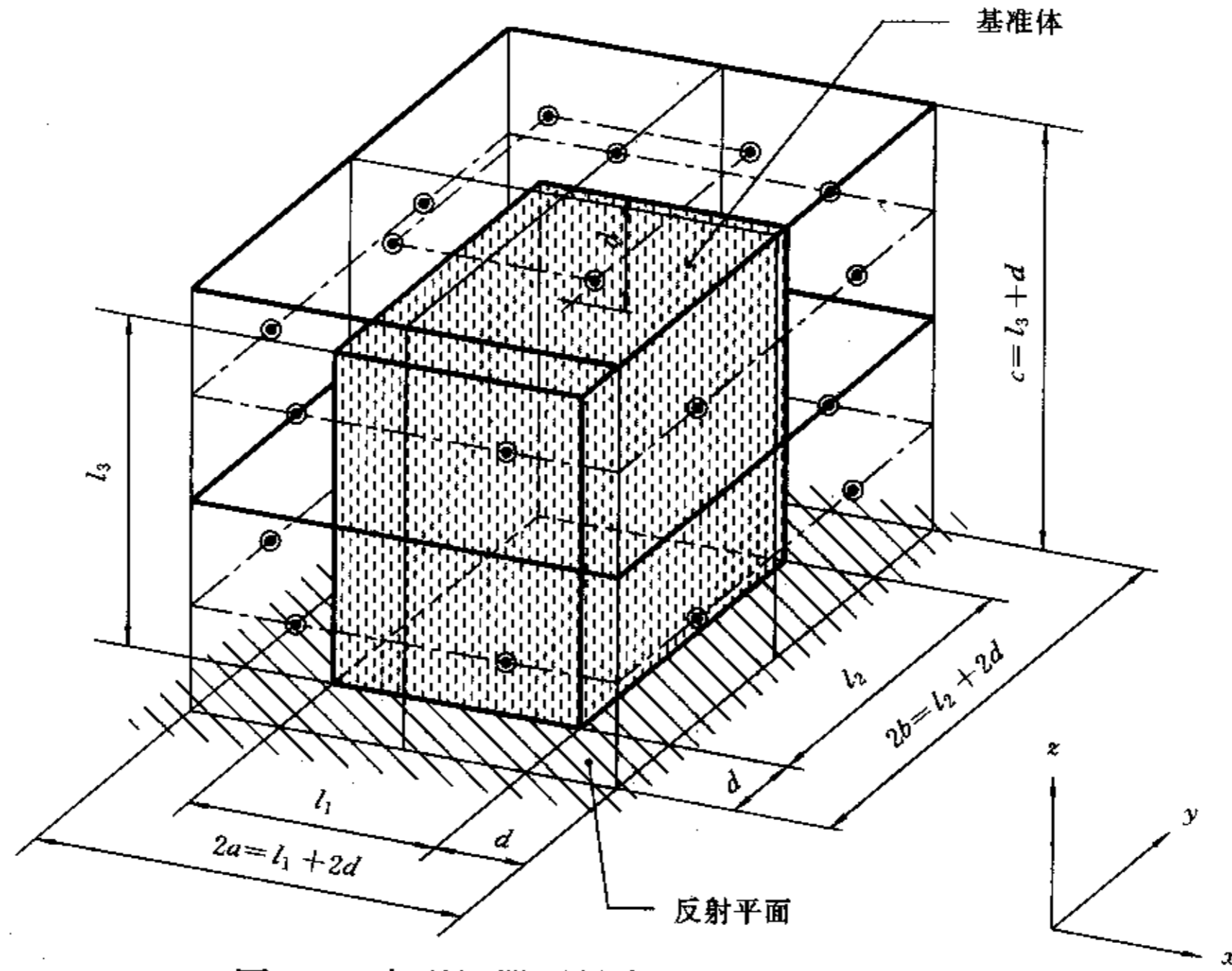
图 C5 中型机器测量表面和传声器位置示例 (d < l_1 \leq 4d, d < l_2 \leq 4d, 2d < l_3 \leq 5d)
